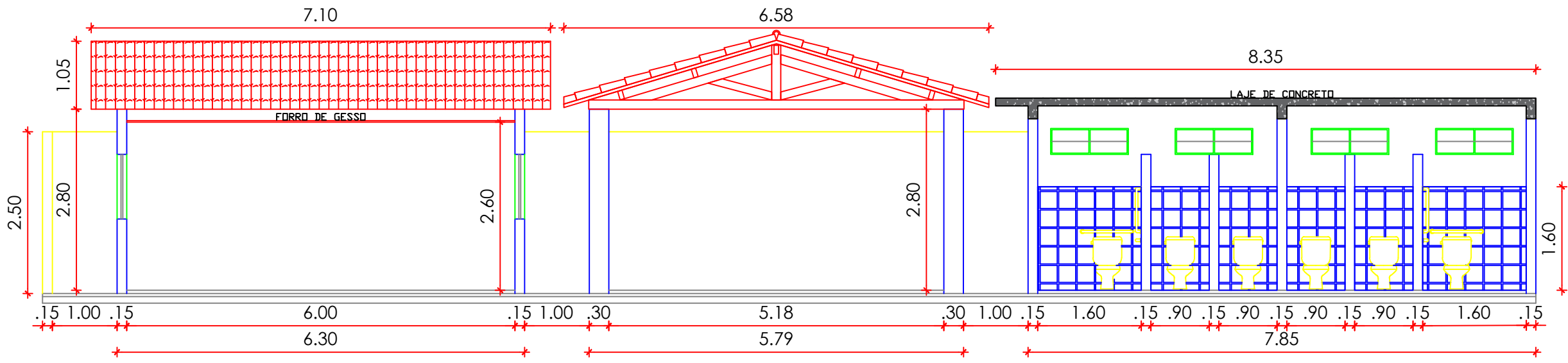
CORTE DD ESC.: 1/75
