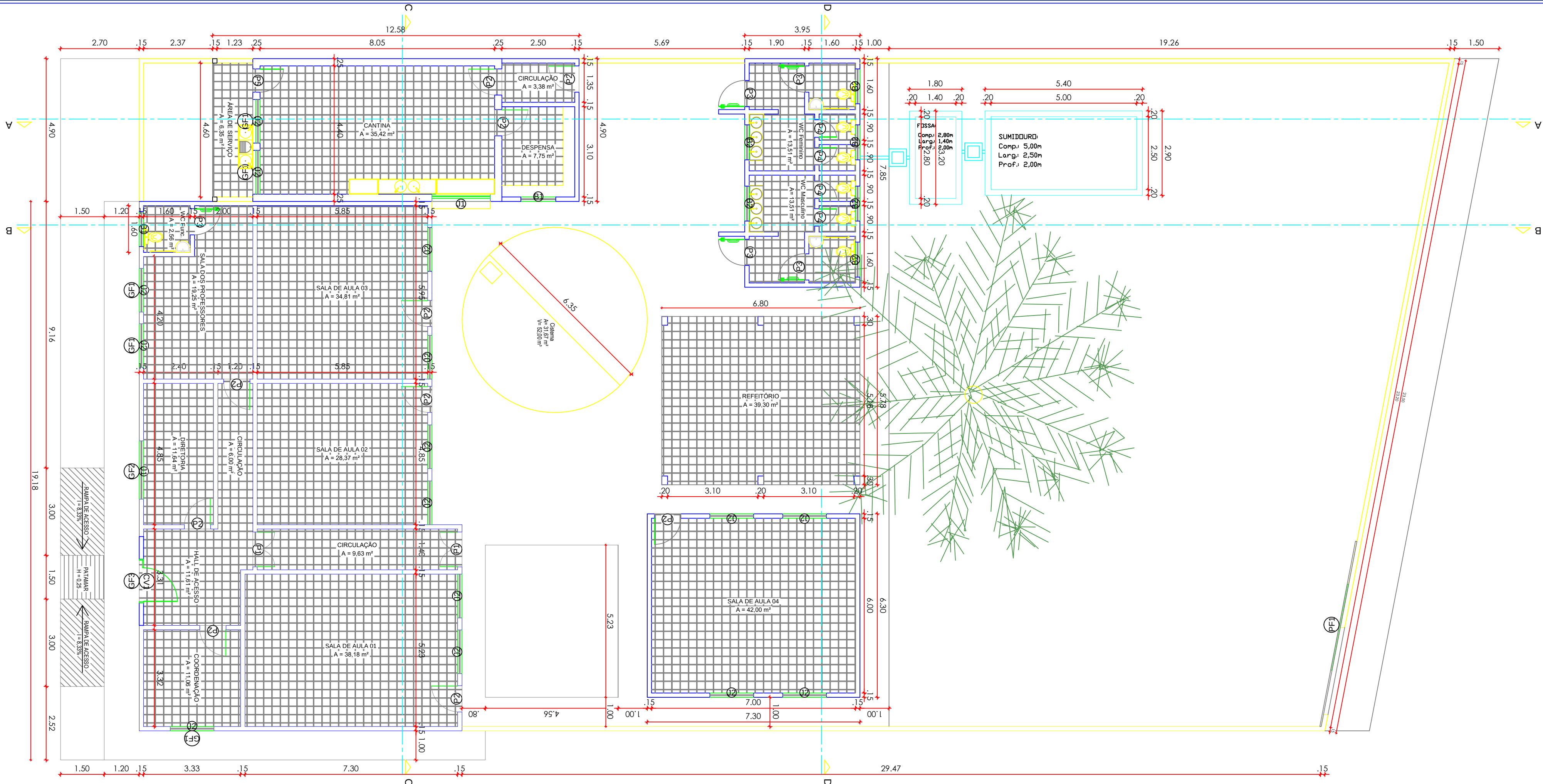
PLANTA BAIXA - PROJETADA ESC.: 1/100
