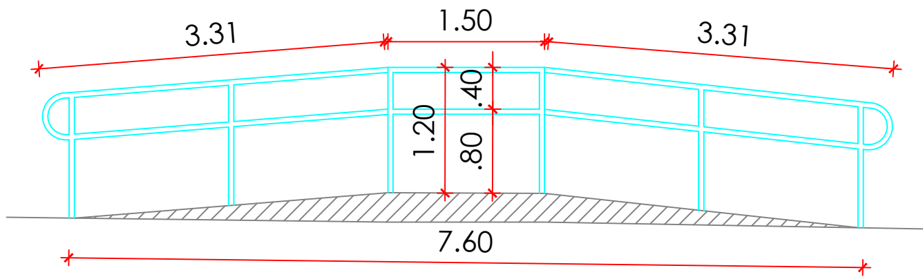
CORRIMÃO - DETALHE ESC.: 1/50
