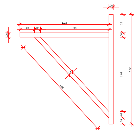
MÃO FRANCESA - LATERAL ESC.: 1/25
