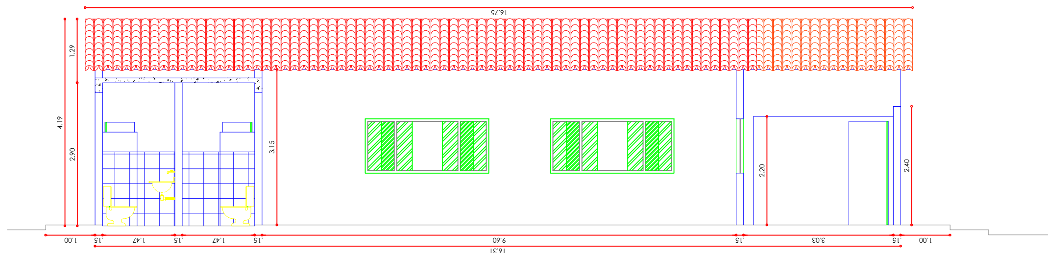
CORTE BB ESC.: 1/75
