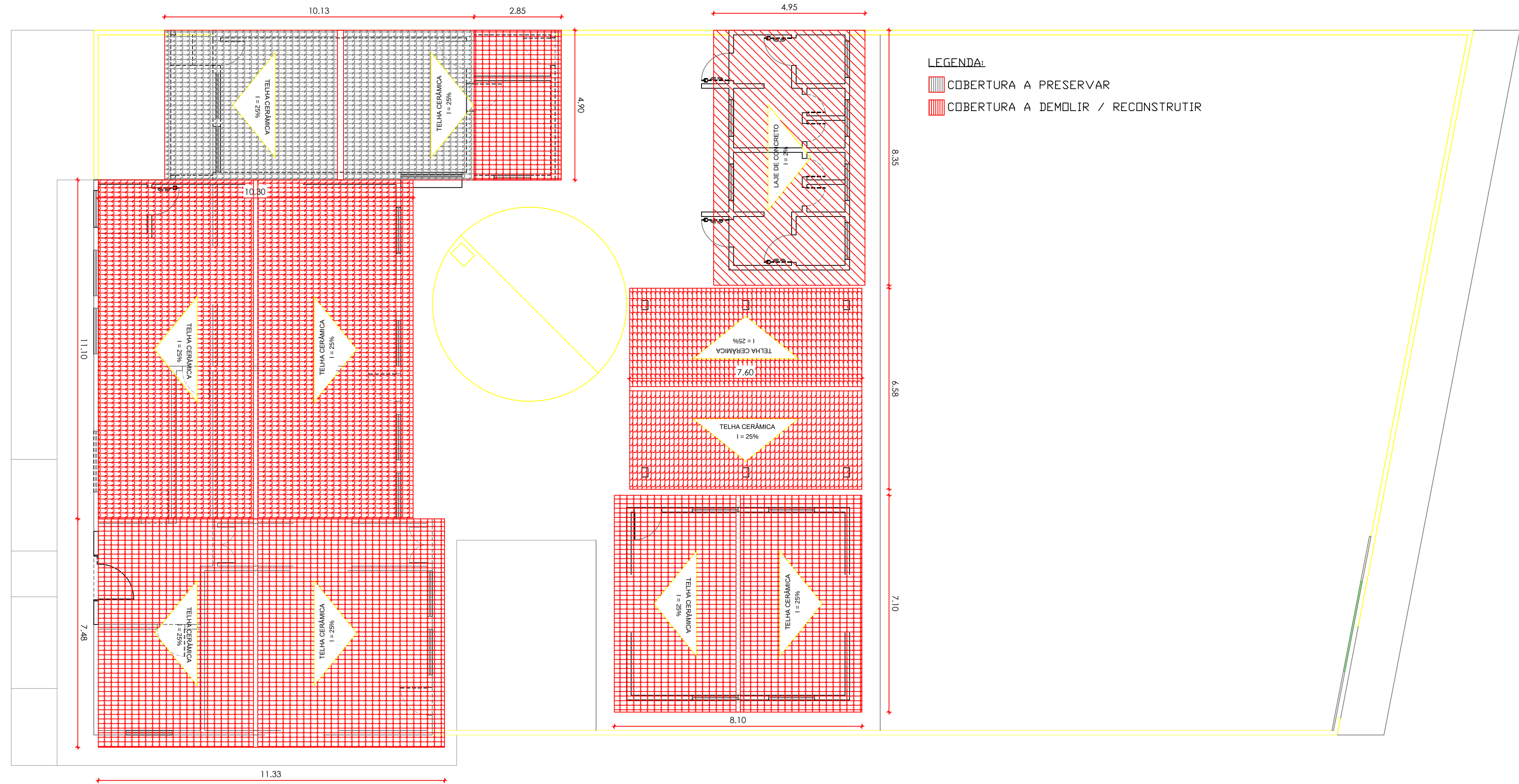
PLANTA DE COBERTURA ESC.: 1/100
