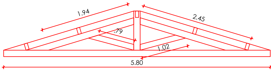
TESOURA ESC.: 1/50
