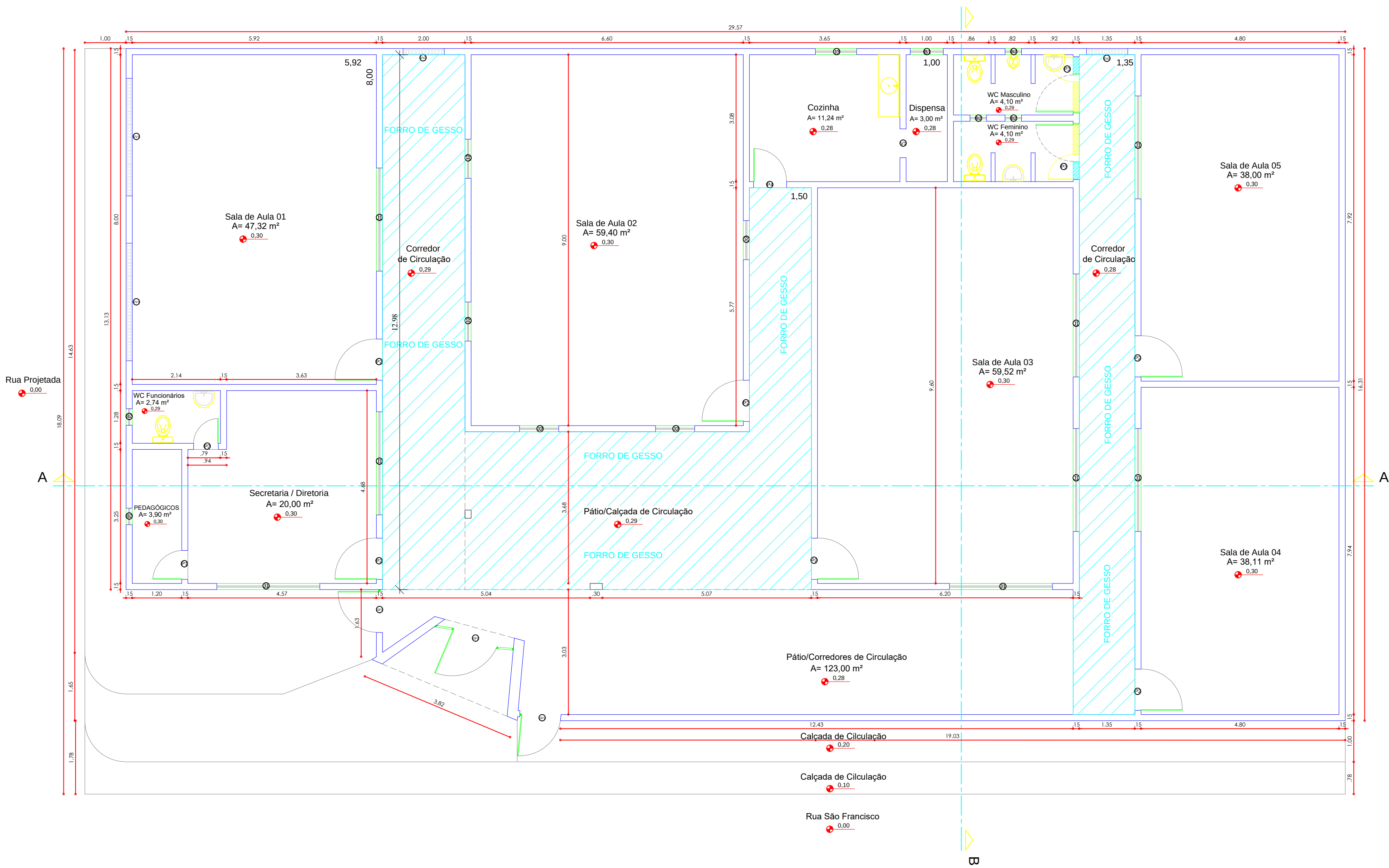
PLANTA BAIXA ESC.: 1/75
