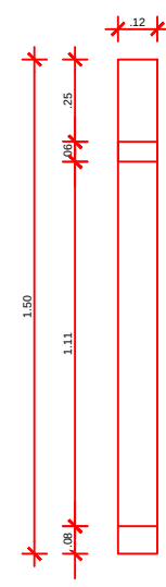
MÃO FRANCESA - FRENTE ESC.: 1/25
